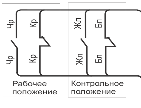
Рисунок В.8 - Схема электрическая принципиальная контактов сигнализации рабочего и контрольного положений выключателей выдвигного исполнения
